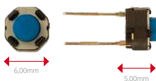
Dimensioni: 6x6x5mm Normalmente aperto Confezione da 10 pz
