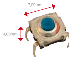
Dimensioni: 7x7x4mm Normalmente aperto Confezione da 10 pz
