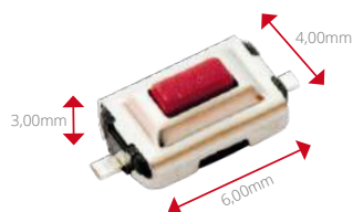
Dimensioni: 6x4x3 mm Normalmente aperto Confezione da 10 pezzi
